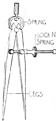
FIG. 41. DIVIDERS.
